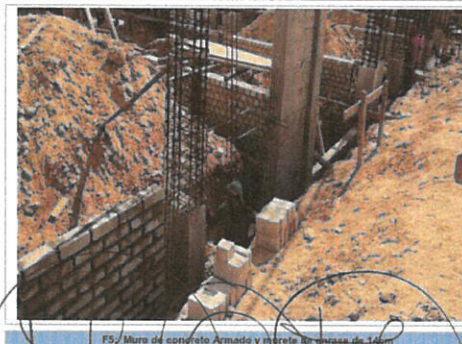
F5: Muro de concreto Armado y murete de enrase de 15cm
